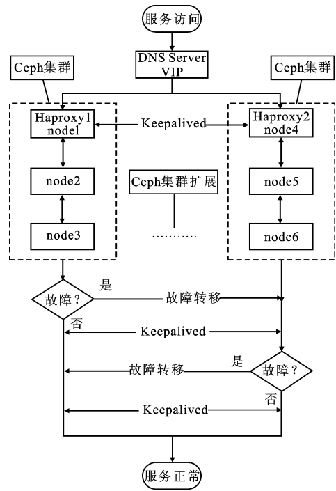
图 4 高可用性设计框架
